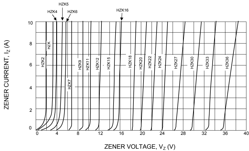
FIG.3 - ZENER CURRENT vs. ZENER VOLTAGE
